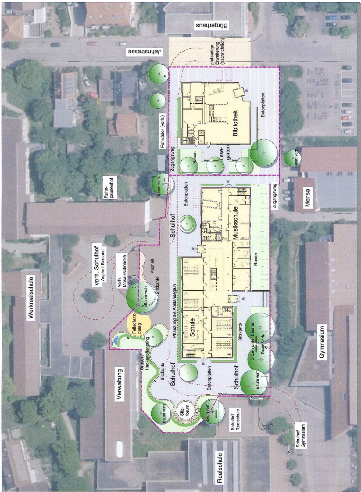
Übersichtsplan
